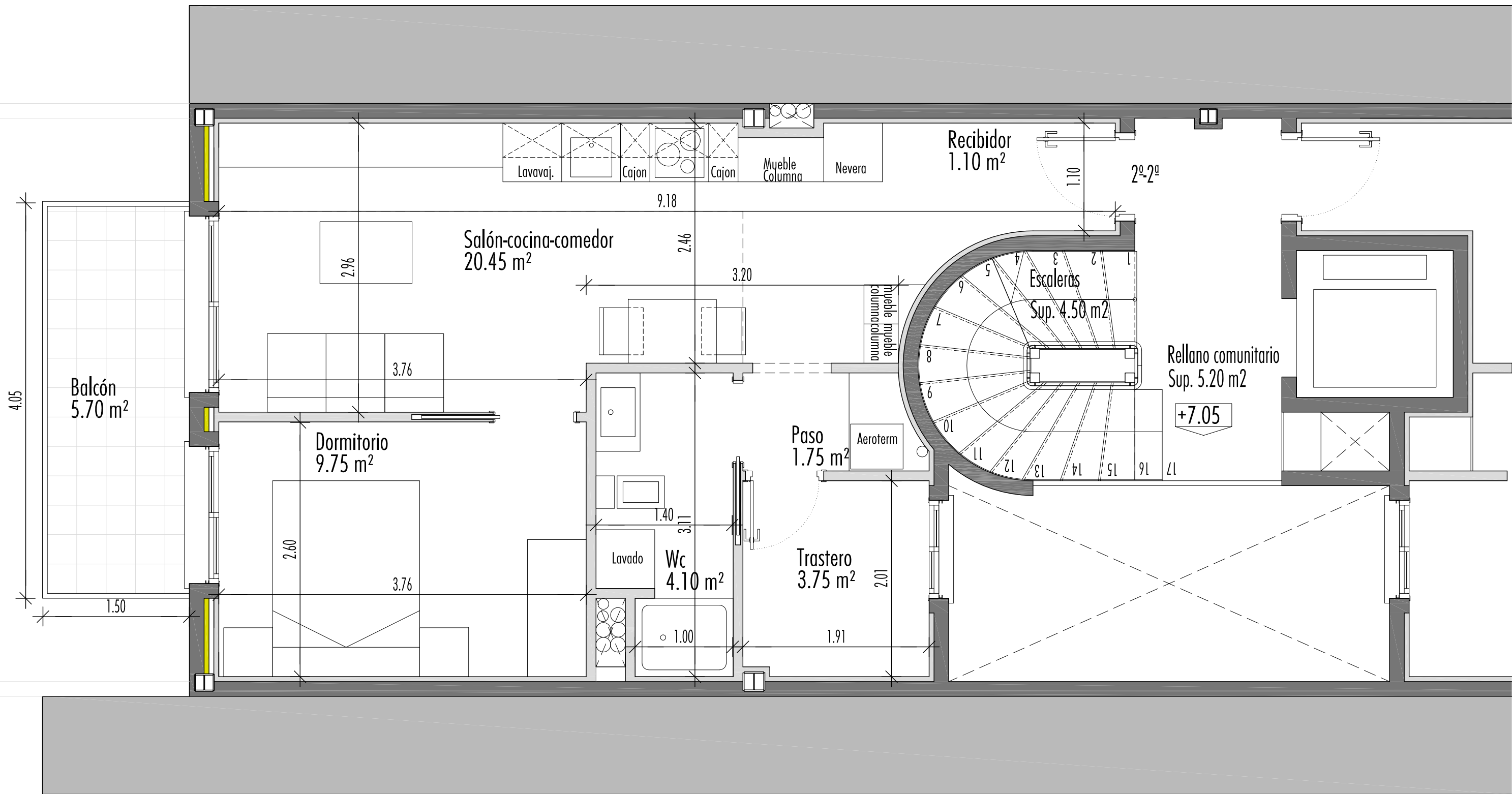
PLANTA 2ª apartamento 2ª
